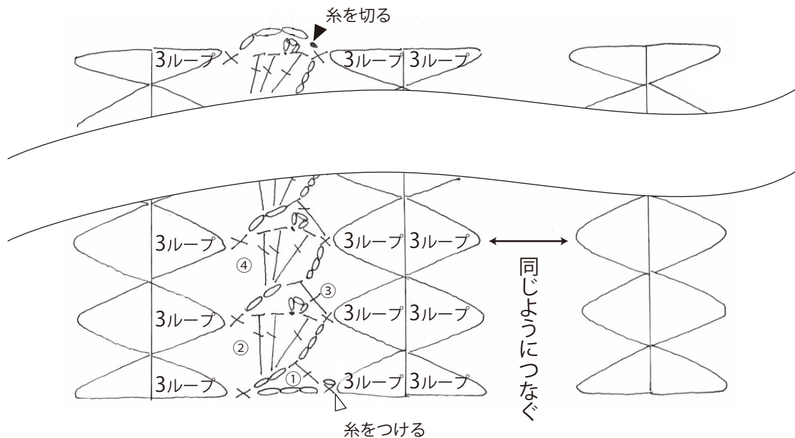
図1 ヘアピンのブレードを3ループずつまとめながらつないでいく。
